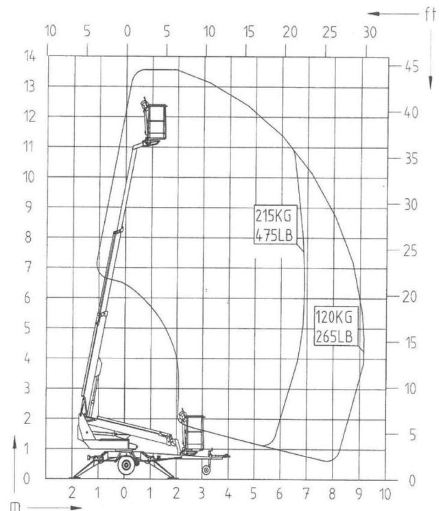
REICHWEITENDIAGRAMM
