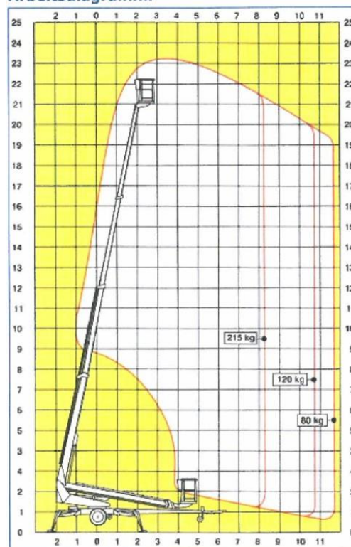
Arbeitsdiagramm:
