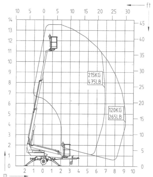
REICHWEITENDIAGRAMM
