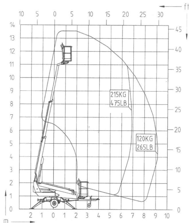
REICHWEITENDIAGRAMM
